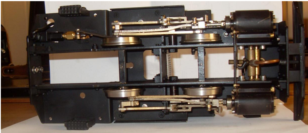
Mechanische voedingspomp
