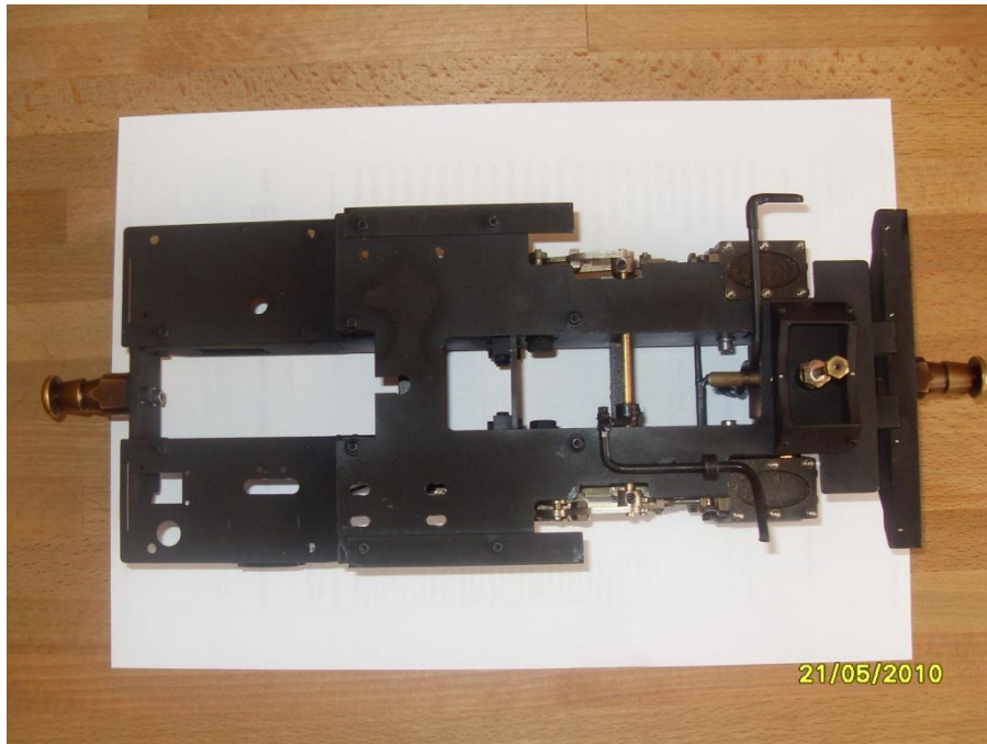
Bediening ontwatering (links) en rijrichting Heusinger (rechts)
