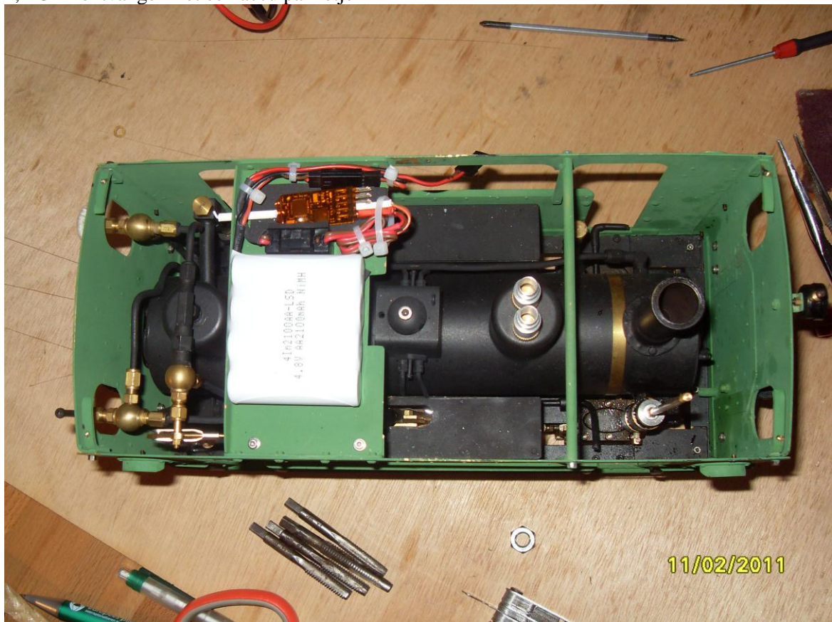
2,4 GHz ontvanger met een accu pakketje
