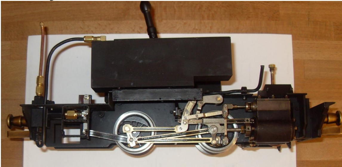
Mechanische voedingspomp
