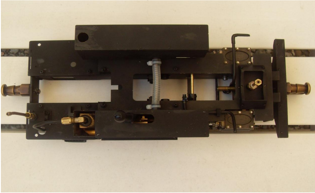
Waterbakken gemonteerd
